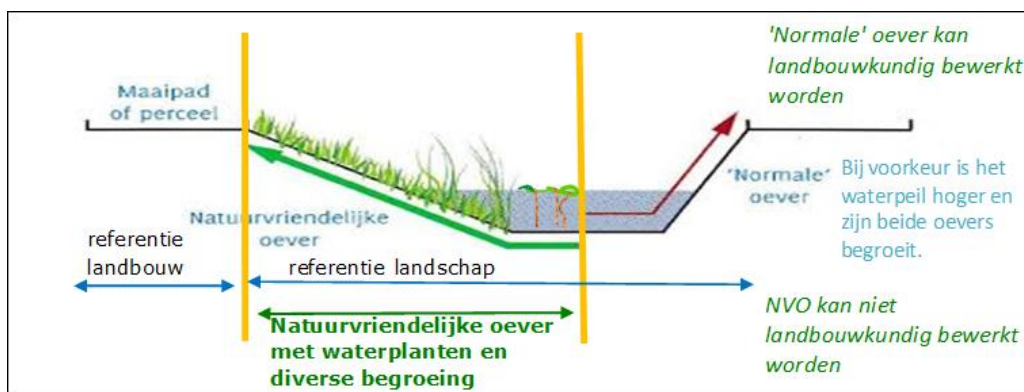
Figuur 1: Tekening natuurvriendelijke oever (NVO) © BoerenNatuur.
